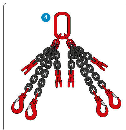
4 4-Sprong + inkortklauwen Lengte: Naar wens Dikte: 8-10-13 mm
