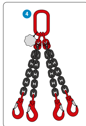
4 4-Sprong Lengte: Naar wens Dikte: 8-10-13 mm
