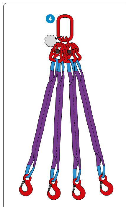
4 4-Sprong + Lengte: Naar wens Bandtype: Naar wens
