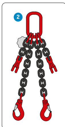
2 2-Sprong + inkortklauwen Lengte: Naar wens Dikte: 8-10-13 mm
