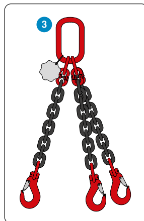
3 3-Sprong Lengte: Naar wens Dikte: 8-10-13 mm
