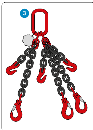
3 3-Sprong + inkort haken Lengte: Naar wens Dikte: 8-10-13 mm
