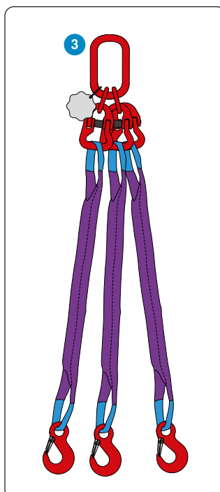
3 3-Sprong + Lengte: Naar wens Bandtype: Naar wens
