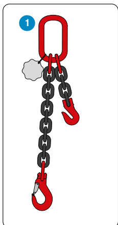
1 Kettingleng + inkort haak Lengte: Naar wens Dikte: 8-10-13 mm
