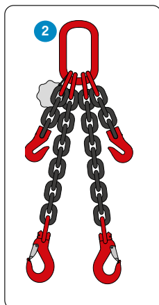
2 2-Sprong + inkort haken Lengte: Naar wens Dikte: 8-10-13 mm
