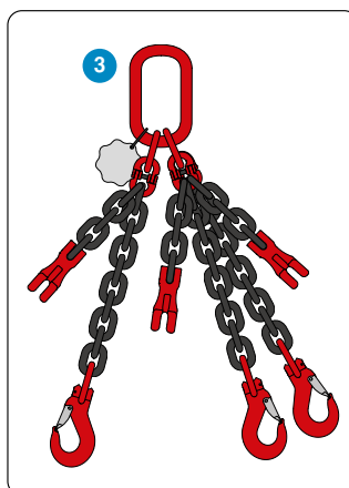
3 3-Sprong + inkortklauwen Lengte: Naar wens Dikte: 8-10-13 mm
