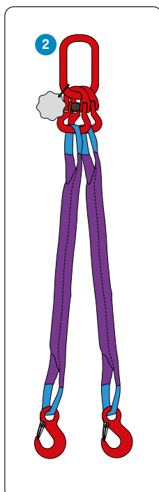
2 2-Sprong + Lengte: Naar wens Bandtype: Naar wens
