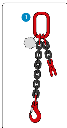
1 Kettingleng + inkortklauw Lengte: Naar wens Dikte: 8-10-13 mm
