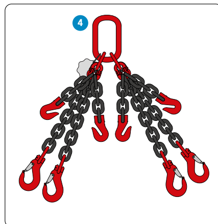
4 4-Sprong + inkort haken Lengte: Naar wens Dikte: 8-10-13 mm
